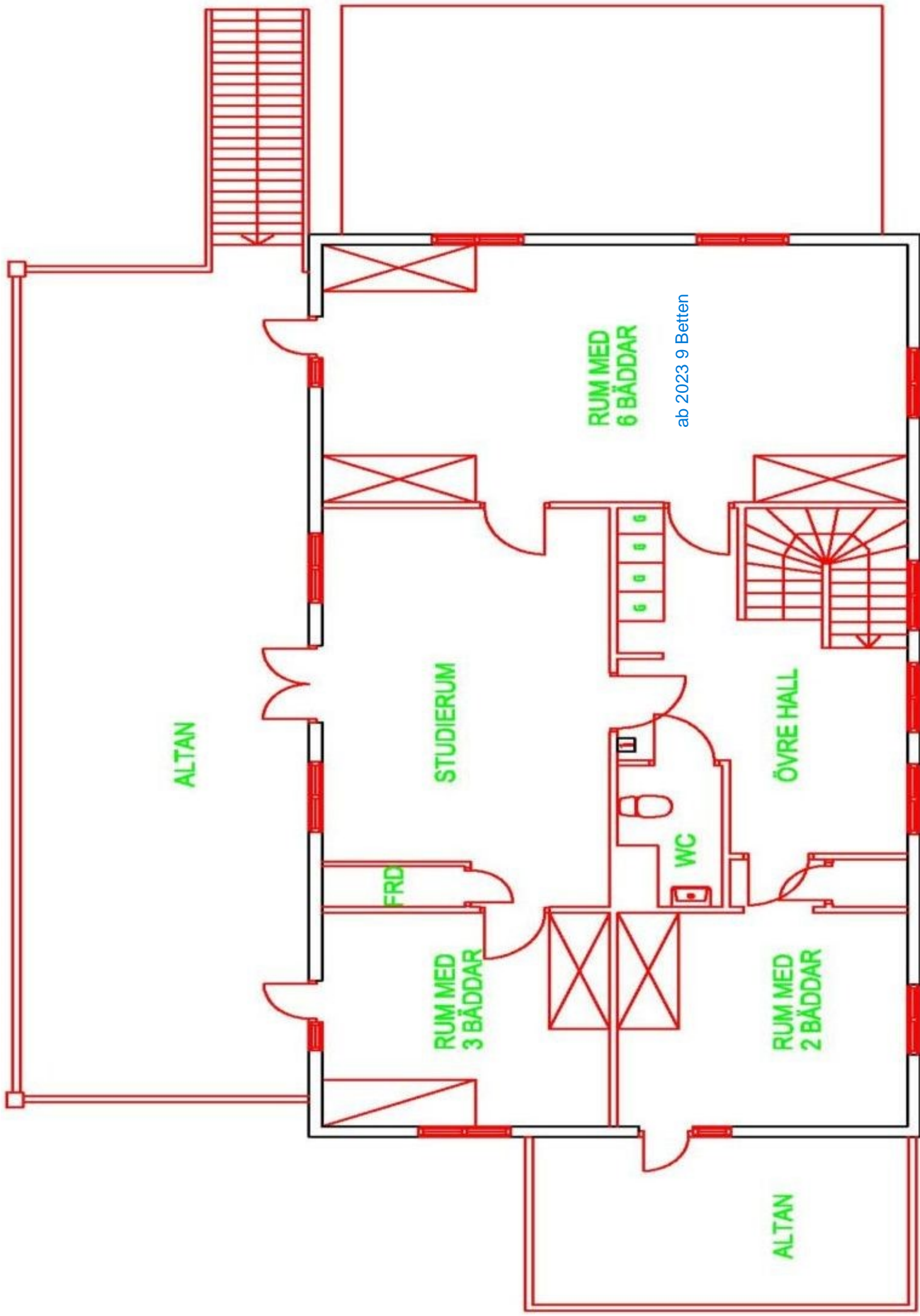
PLAN VÅN 2
